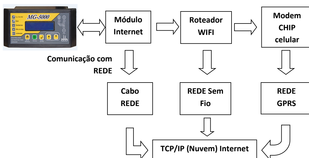
Diagrama de Blocos – Sistema de Comunicação INTERNET
